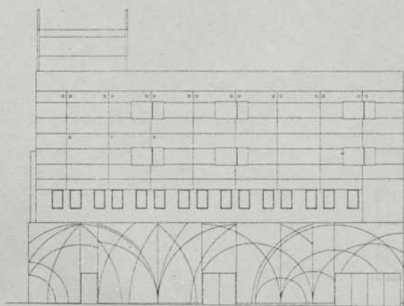
Façade nord.
