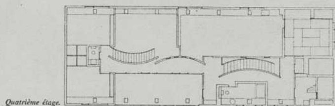
Quatrième étage.
